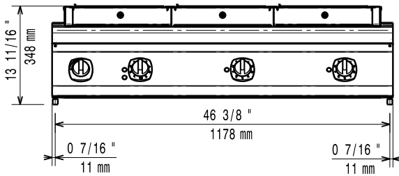
Front aanzicht
